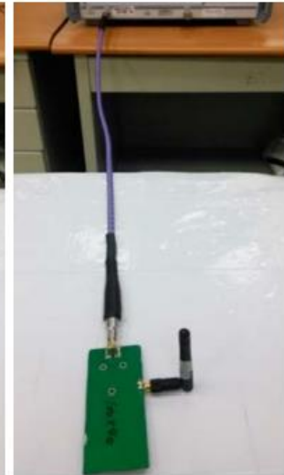
Antenna R/A
